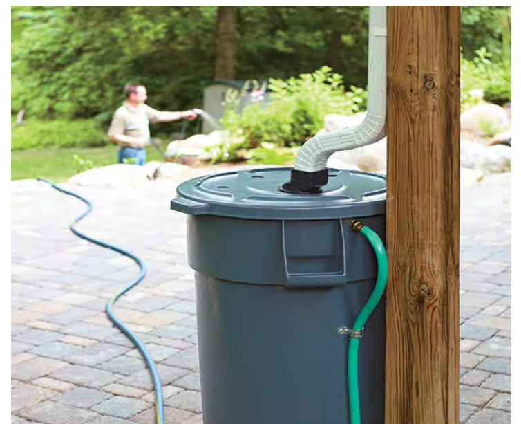
Coleta de água das chuvas em residência - arquitetura sustentável - Imagem do Portal Eco Debate
